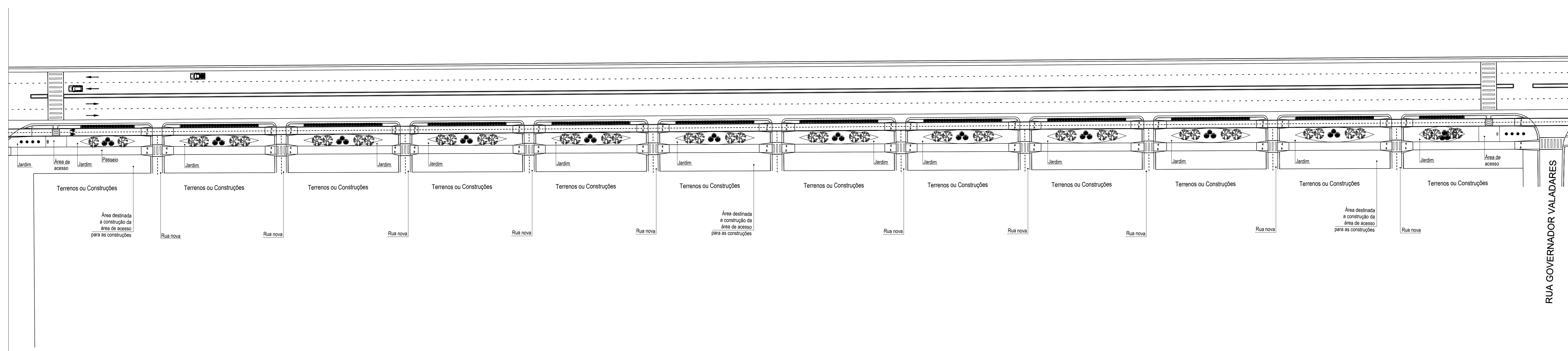
PLANTA BAIXA - Trecho 02 ESC. 1/500
